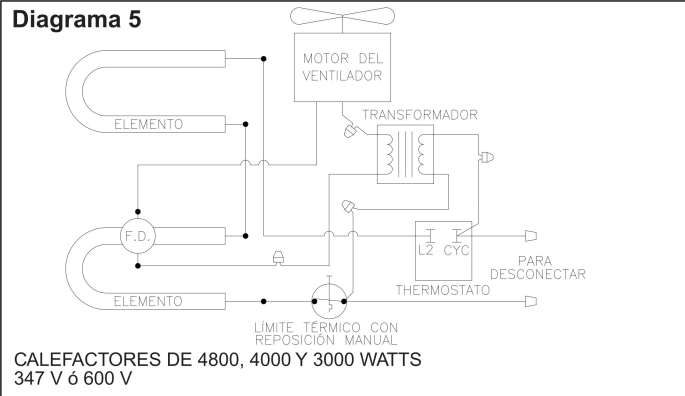
DIAGRAMA DE CABLEADO PARA CALENTADORES DE PARED TRIFÁSICOS
