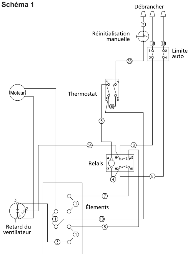
SCHÉMA DE CÂBLAGE POUR APPAREILS DE CHAUFFAGE MURAL TRIPHASÉS
