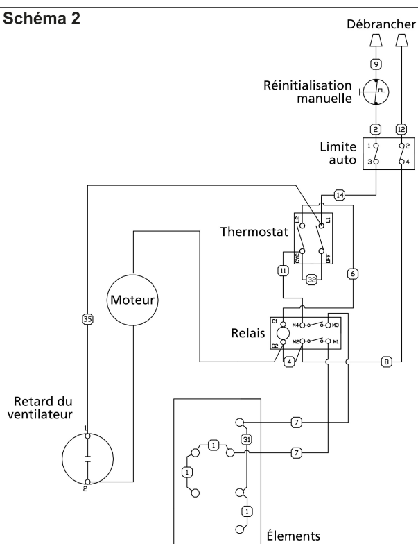
SCHÉMA DE CÂBLAGE POUR APPAREILS DE CHAUFFAGE MURAL MONOPHASÉS 208V, 4800W
